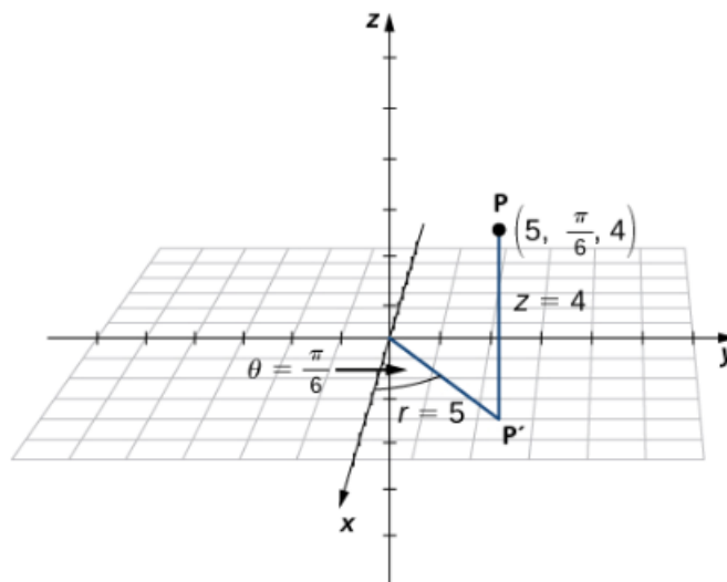
Figura 3: Libretexts - Exemplo das coordenadas cilíndricas de um ponto
