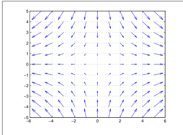
Campo vetorial (3x, -3y) .
