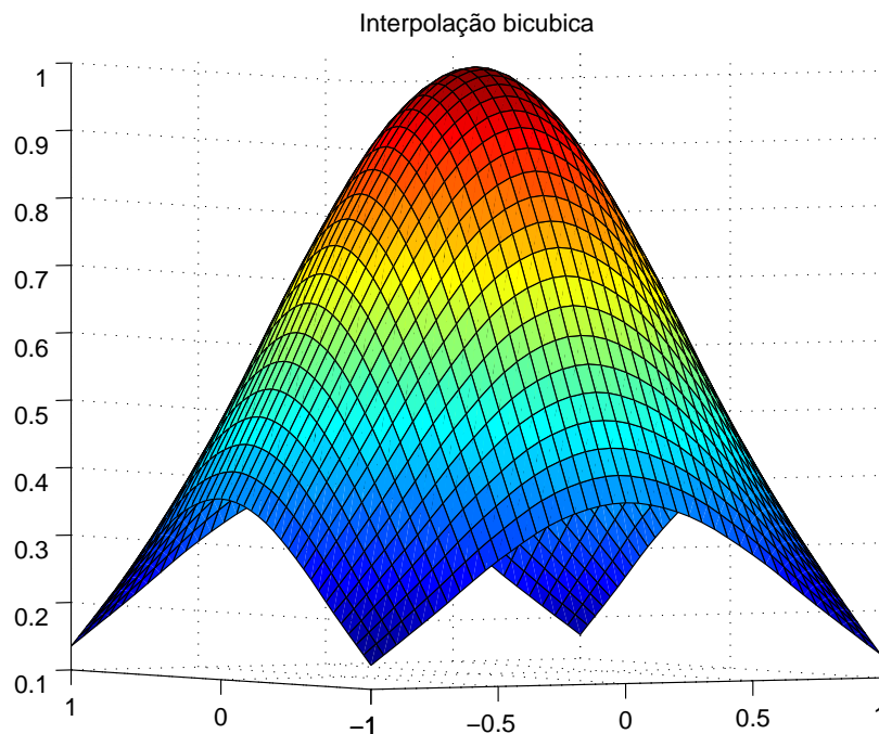
Figura 6: Interpolação bicúbica
